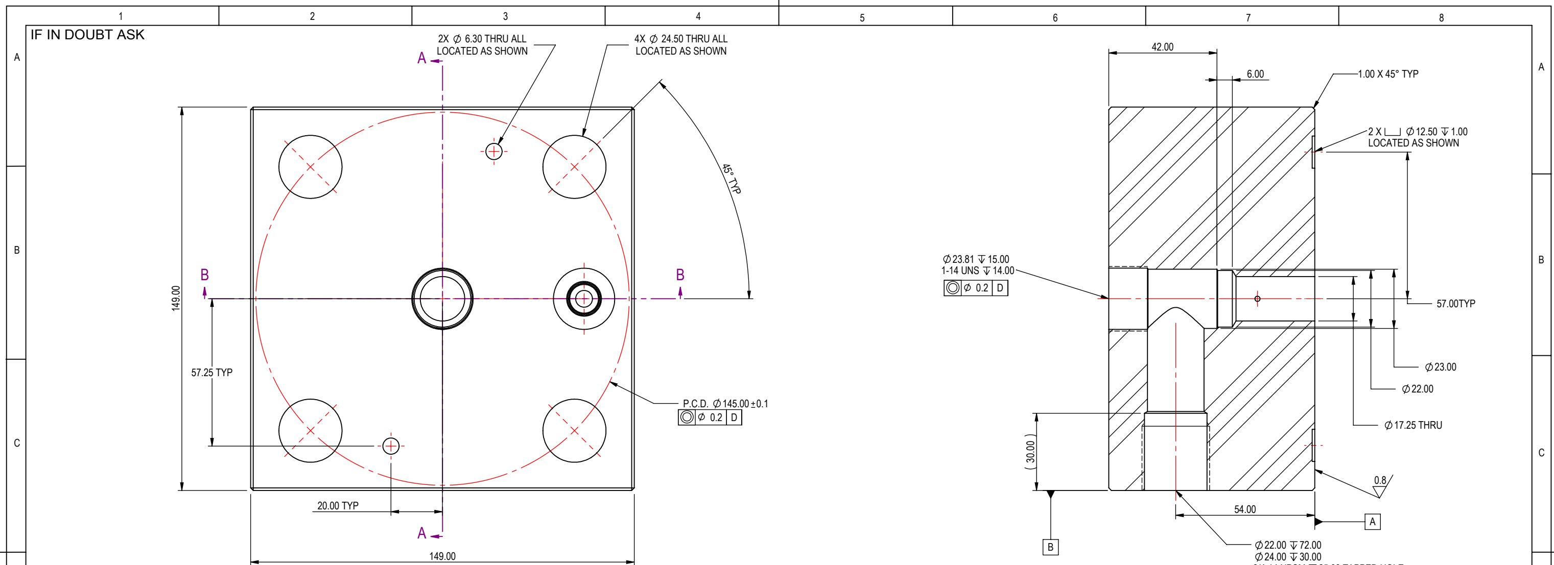
SECTION A-A
