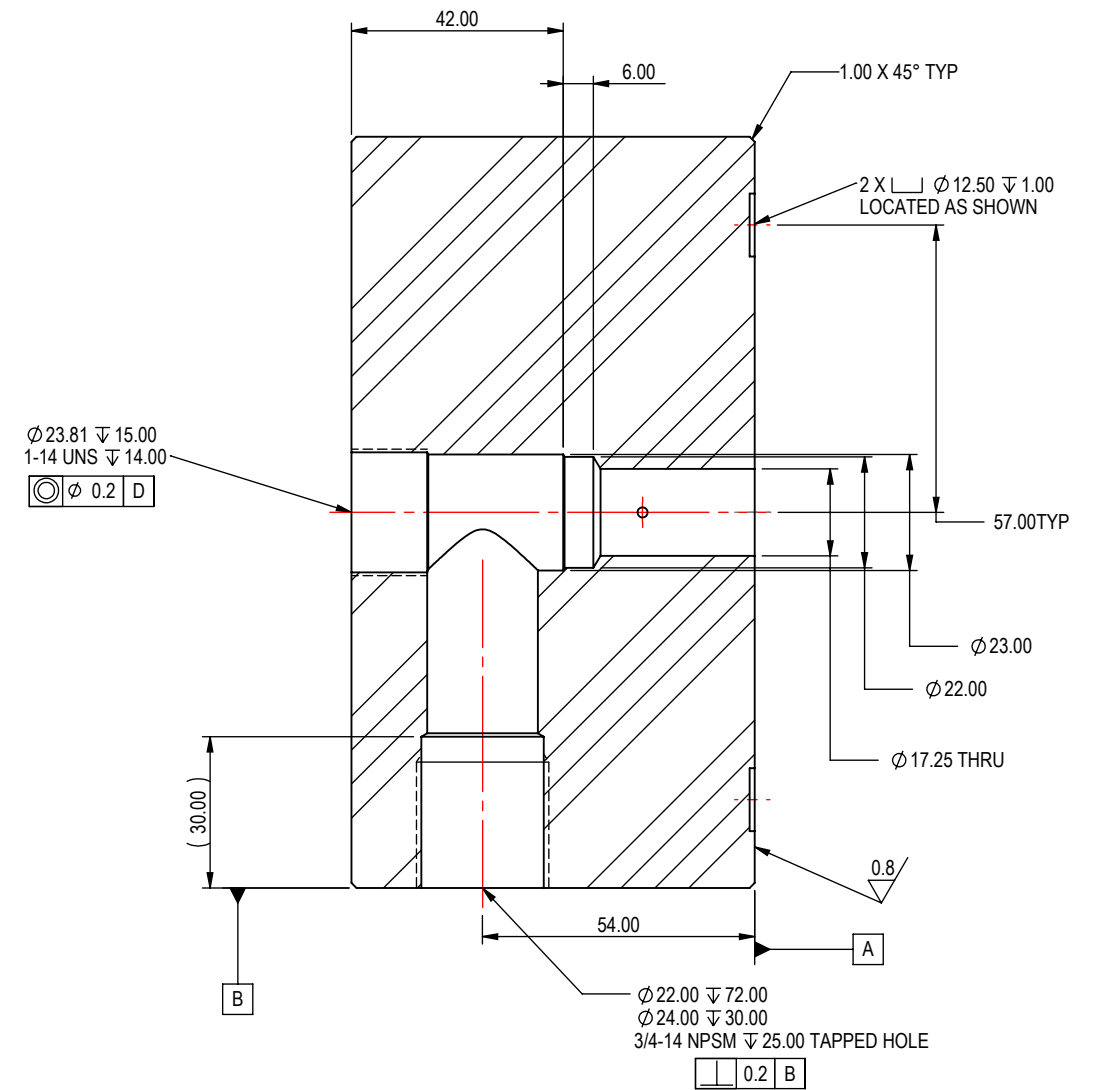
SECTION A-A
